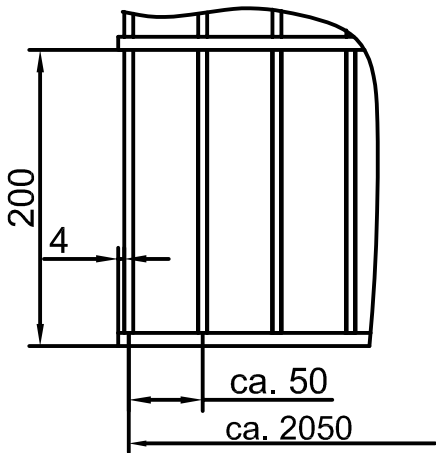
Einzelheit Z
